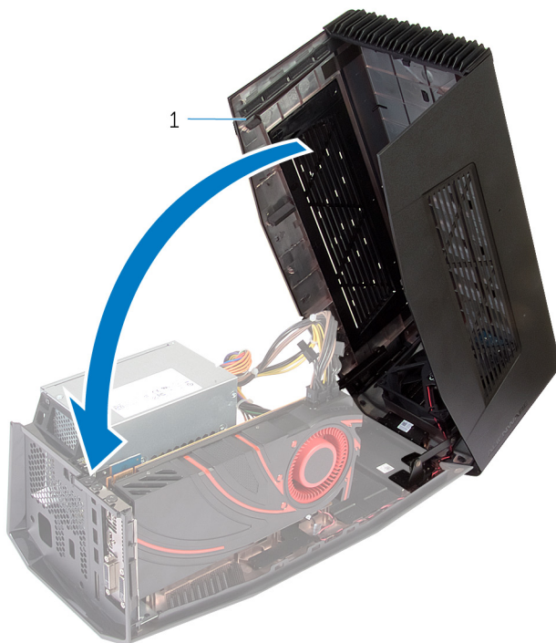
1 Abdeckung
